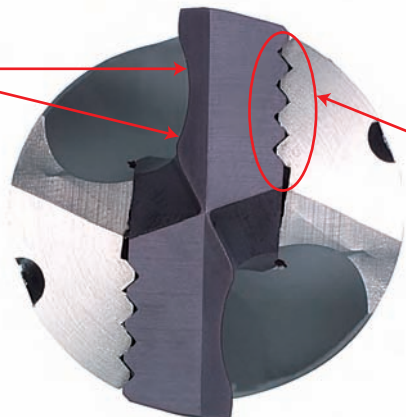
切削刃形状
